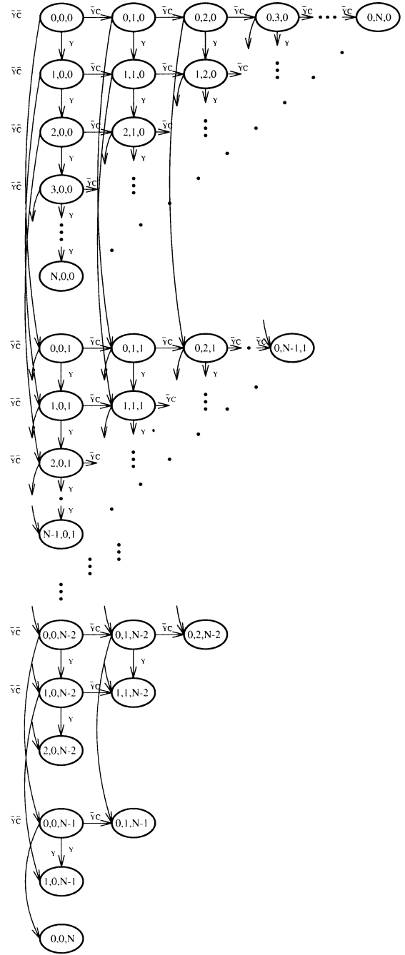
Fig. 4. CQL model.
